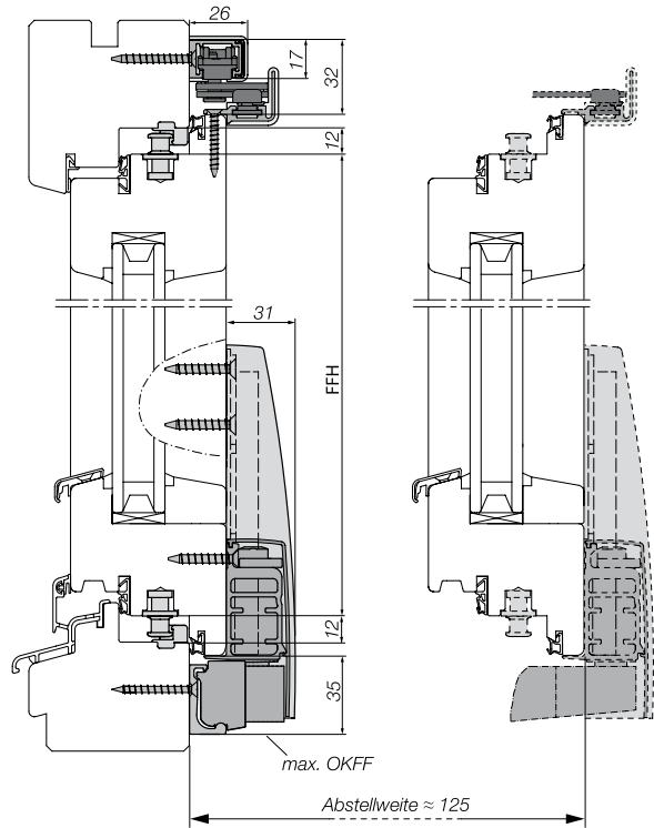
Höhenschnitt Holz
