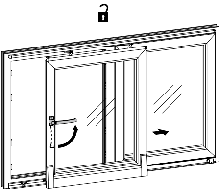
Schiebestellung
