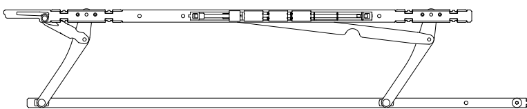
26 Gleitschere
