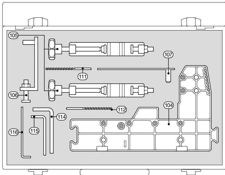
Lehrenkoffer
