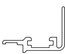
38 Halteschiene 13
